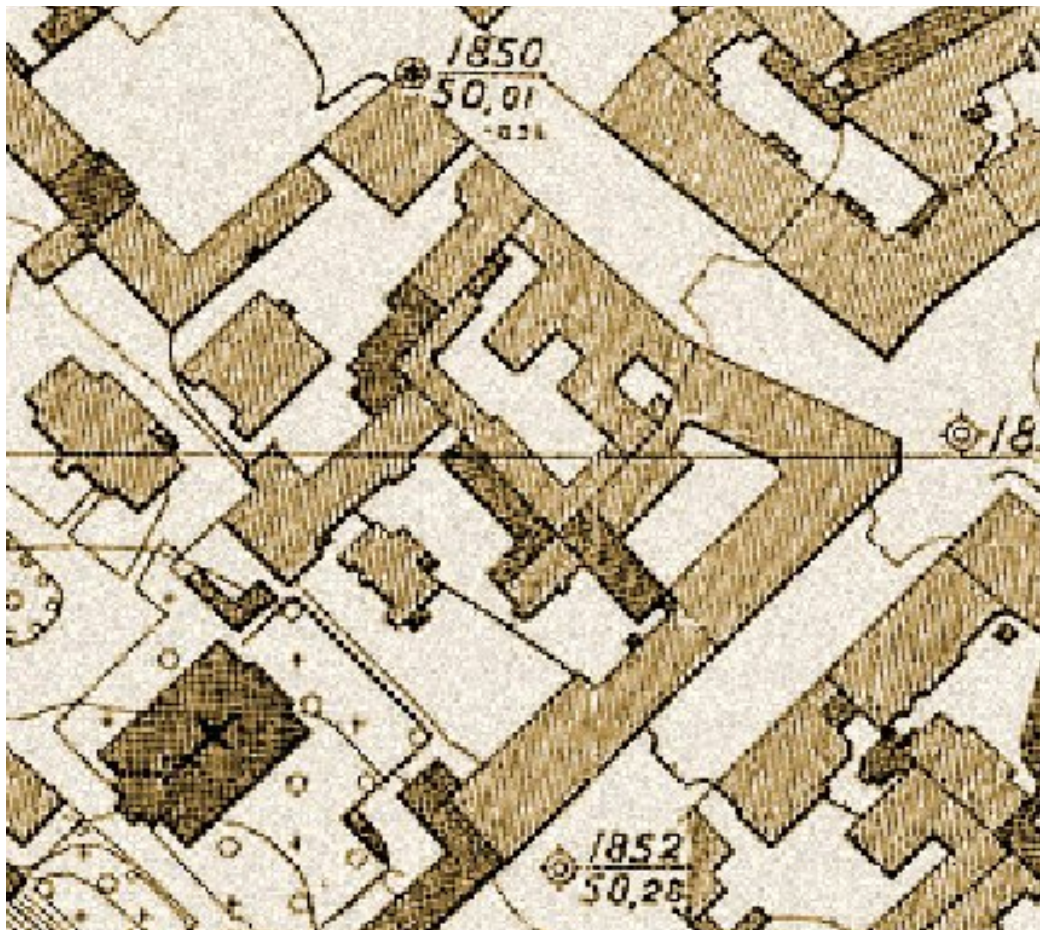
Подол. Топографический план Киевского Округомгоспу. Лист 121. 1923–1925 гг. Масштаб 25 саж. в дюйме. Фрагмент [з колекції М.А. Кадомської]
