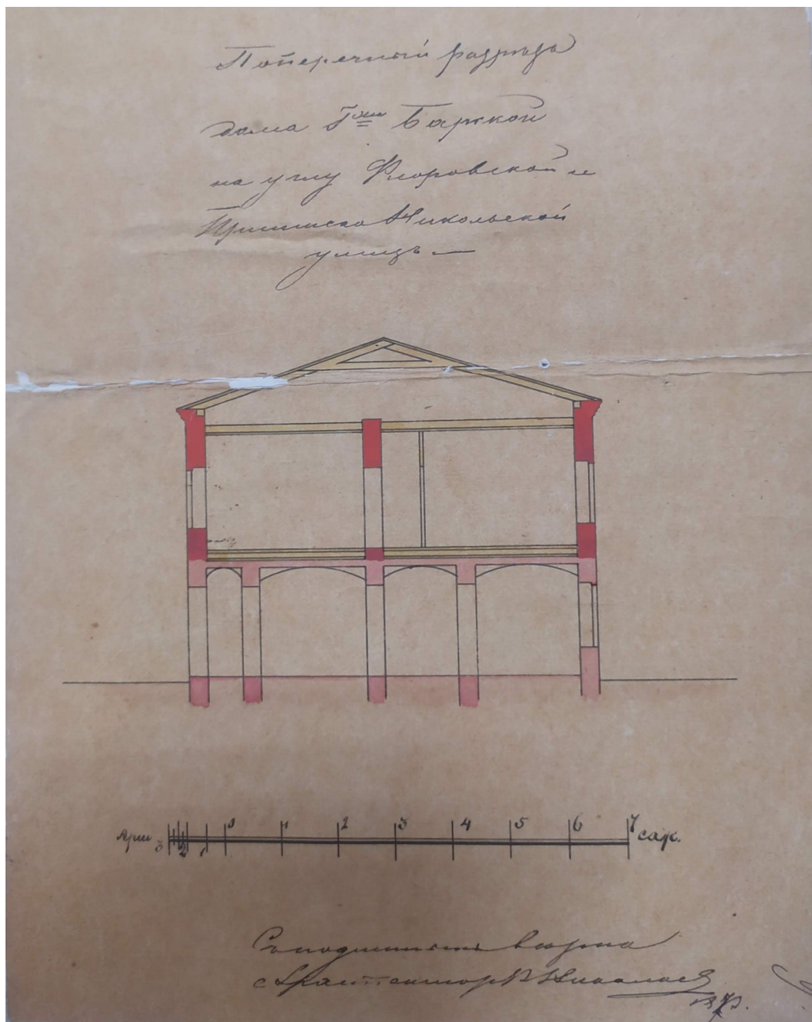
«Поперечный разрез дома Г жи Барской на углу Фроловской и Притиска Никольской улицъ. Архитекторъ В. Николаевъ». 1875 г.
